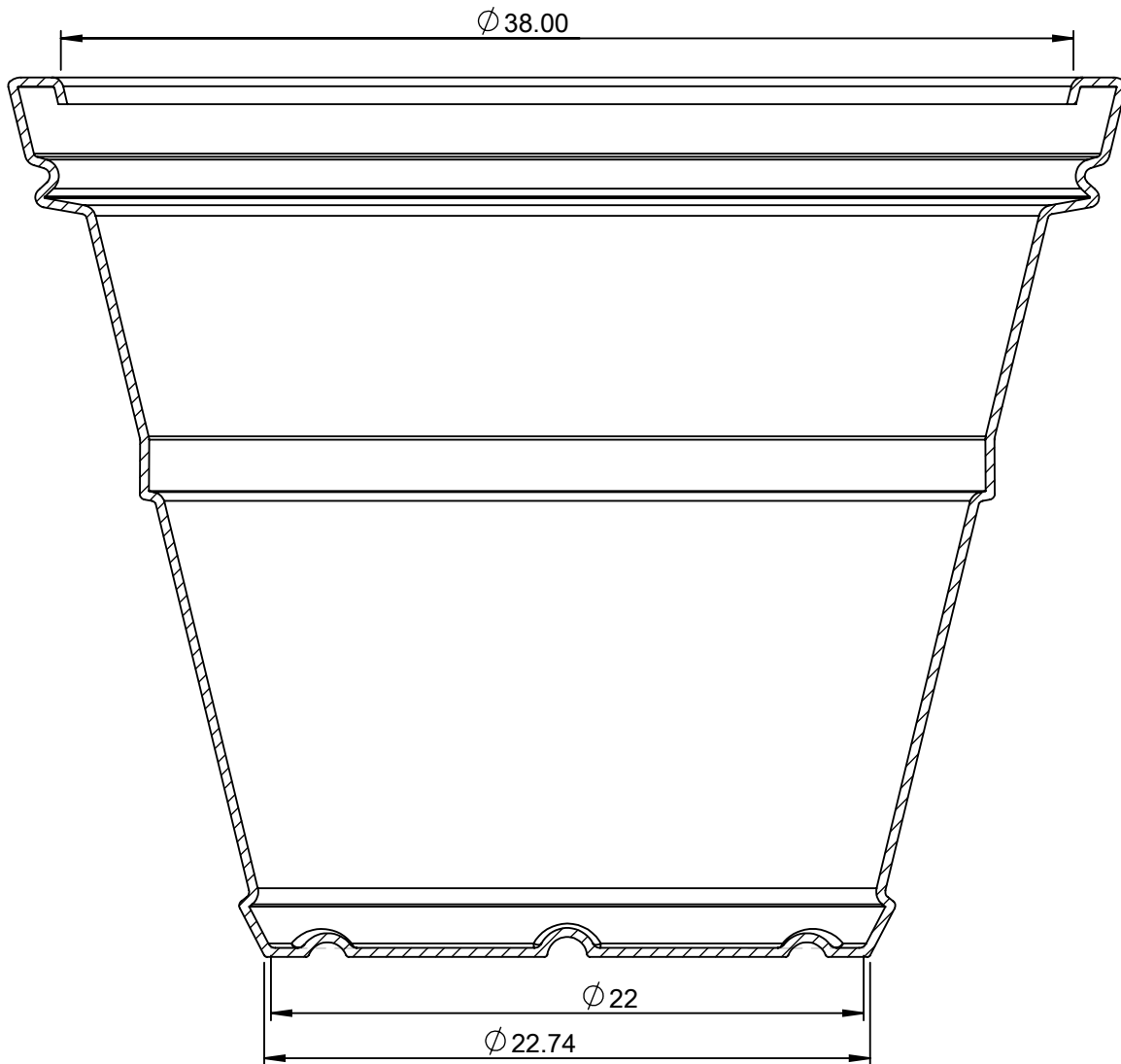
SECTION A-A
