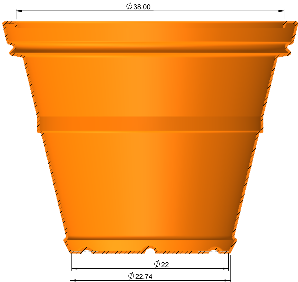
SECTION A-A
